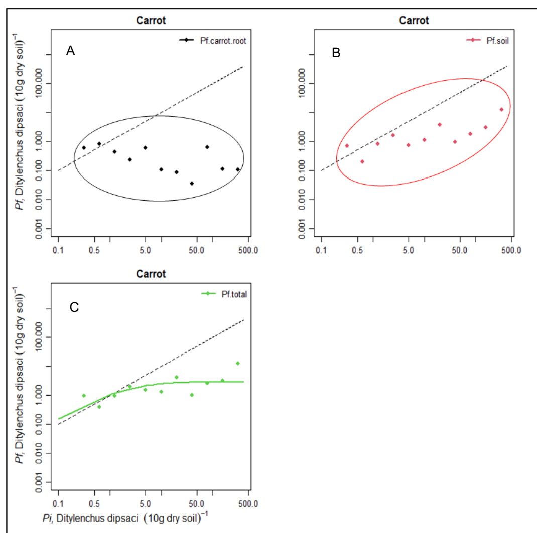
Figuur 6.1 Relatie tussen de begin- ( P_i ) en einddichtheid ( P_f ) van stengelaaltjes 17 weken na inoculatie van peen. A) stengel en wortel, B) grond en C) totaal. De stippellijn geeft de situatie weer waarin de P_f gelijk is aan de P_i .
