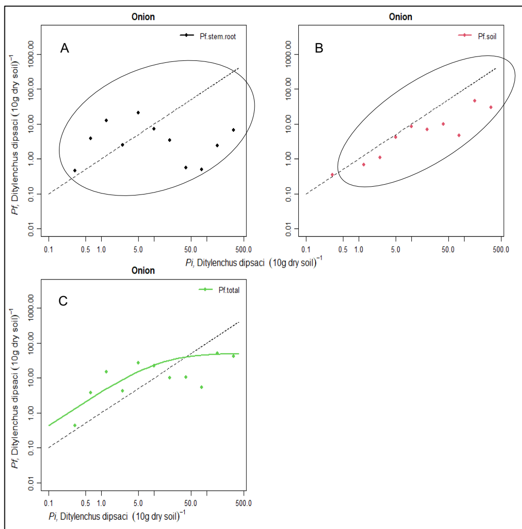
Figuur 6.2 Relatie tussen de begin- ( P_i ) en einddichtheid ( P_f ) van stengelaaltjes 17 weken na inoculatie van ui. A) stengel en wortel, B) grond en C) totaal. De stippellijn geeft de situatie weer waarin de P_f gelijk is aan de P_i .
