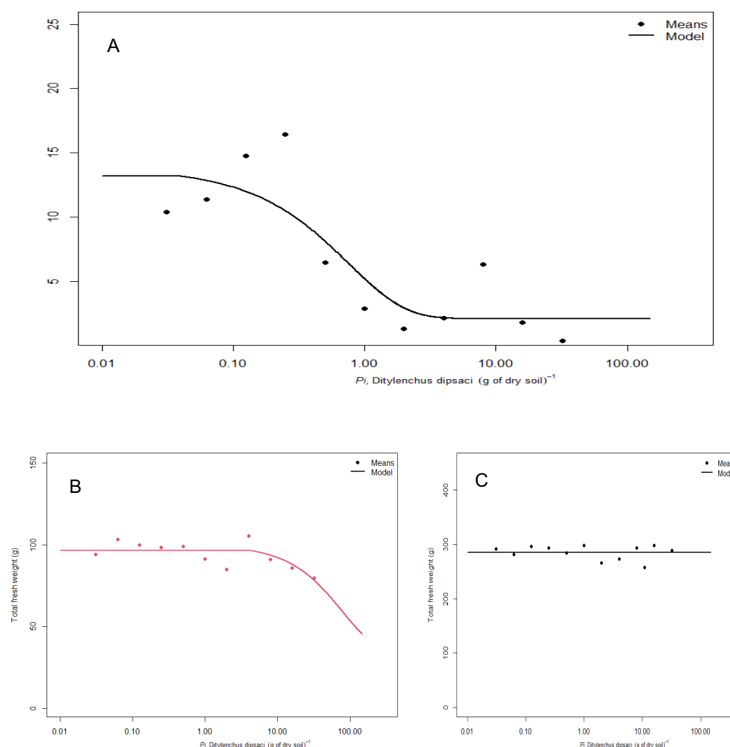
Figuur 6.4 Relatie tussen de begindichtheid van stengelaaftjes en het totaal versgewicht (g) van de plant 17 weken na inoculatie van A) ui, B) peen en C) veldboon.
